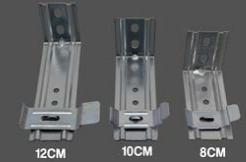
L AYAK PERDE APARATI P-0018 RENK SEÇENEKLERİ : Metal ÜRÜN BOYUTLARI : 8cm,10cm,12cm
